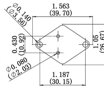
TO-3
